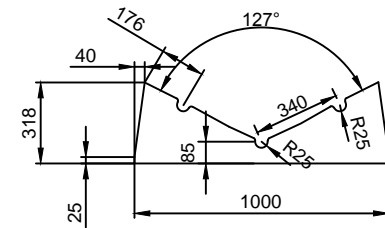
B-B
