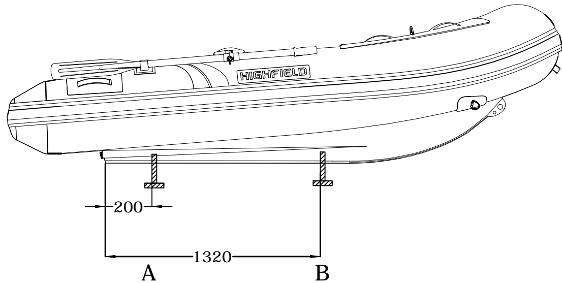
LONGITUDINAL PROFILE
